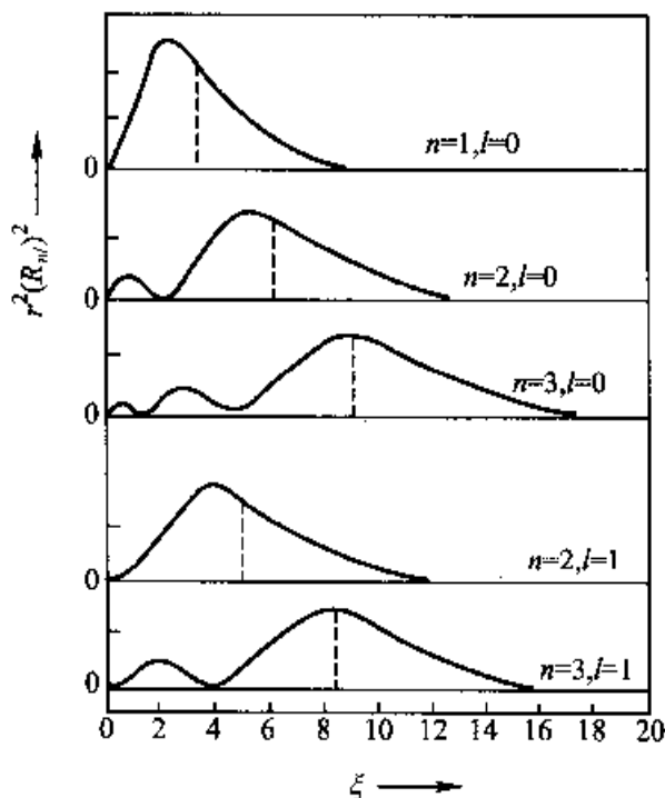
图 5-4 径向概率分布
