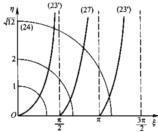
图 2-5 三个圆弧相当于 \frac{2mV_0a^2}{\hbar^2} 分别等于 1, 4, 12
