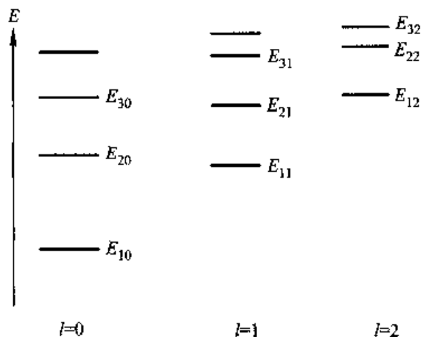
图 5-1 中心力场能级示意图
